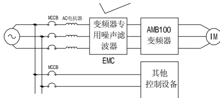
3-5 噪声滤波器的正确设置
