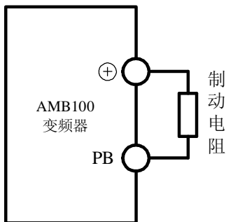
图 9-1 制动电阻的安装
