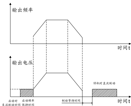
图 5-9 直流制动示意图
