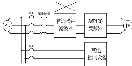
3-5 噪声滤波器的正确设置
