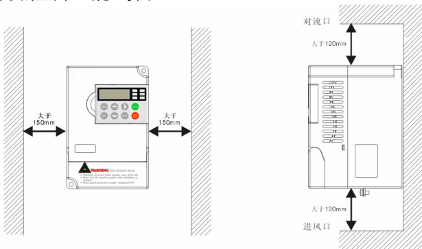
图 2-2 AMB100 变频器安装方向和空间
