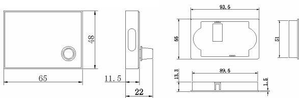
11KW-132KW 规格外型尺寸
