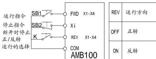
图 5-5 3 线制顺序控制模式 1
