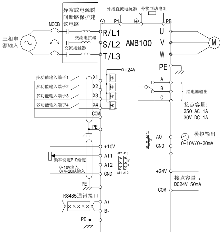
图 3-2-2 AMB100 (11-400KW) 变频器连接图
