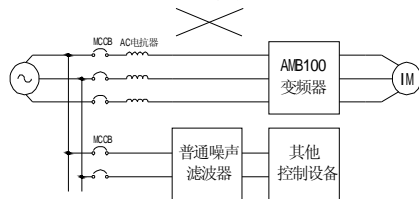
图 3-6 噪声滤波器的错误设置
