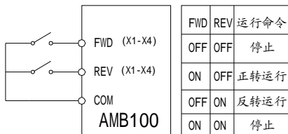
图 5-3 2 线制顺序控制 1
