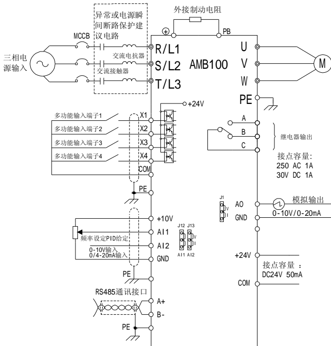
图 3-2-1 AMB100 (0.4-7.5KW) 变频器连接图
