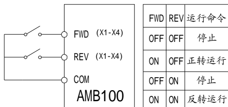
图 5-4 2 线制顺序控制 2
