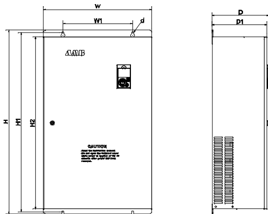
160KW 及以上规格外型尺寸
