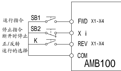
图 5-6 3 线制顺序控制模式 2
