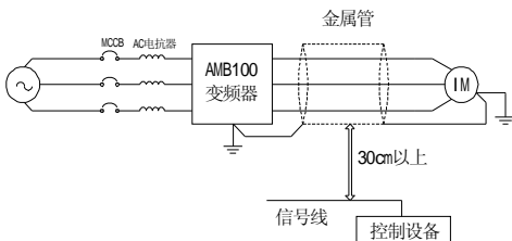
图 3-8 传导干扰对策
