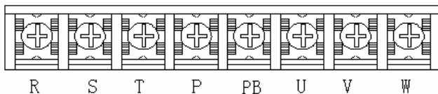
220V/380V(0.4-7.5KW)主回路端子
