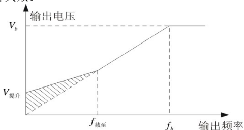
图 5-12 手动转矩提升示意图
