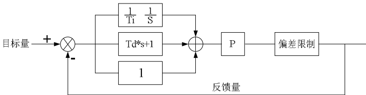
图 5-18 过程 PID 原理框图
