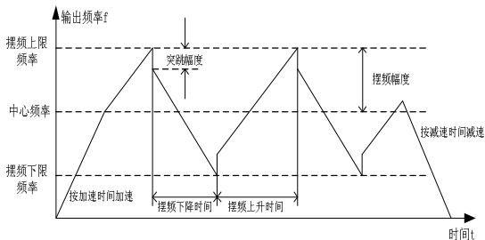
图 5-15 摆频运行示意图
