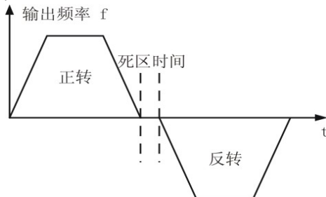
图 5-10 正反转死区时间示意图
