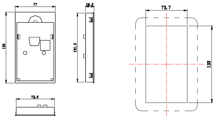
160KW 及以上规格外型尺寸
