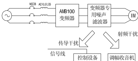
图 3-7 输出侧噪声滤波器的安装
